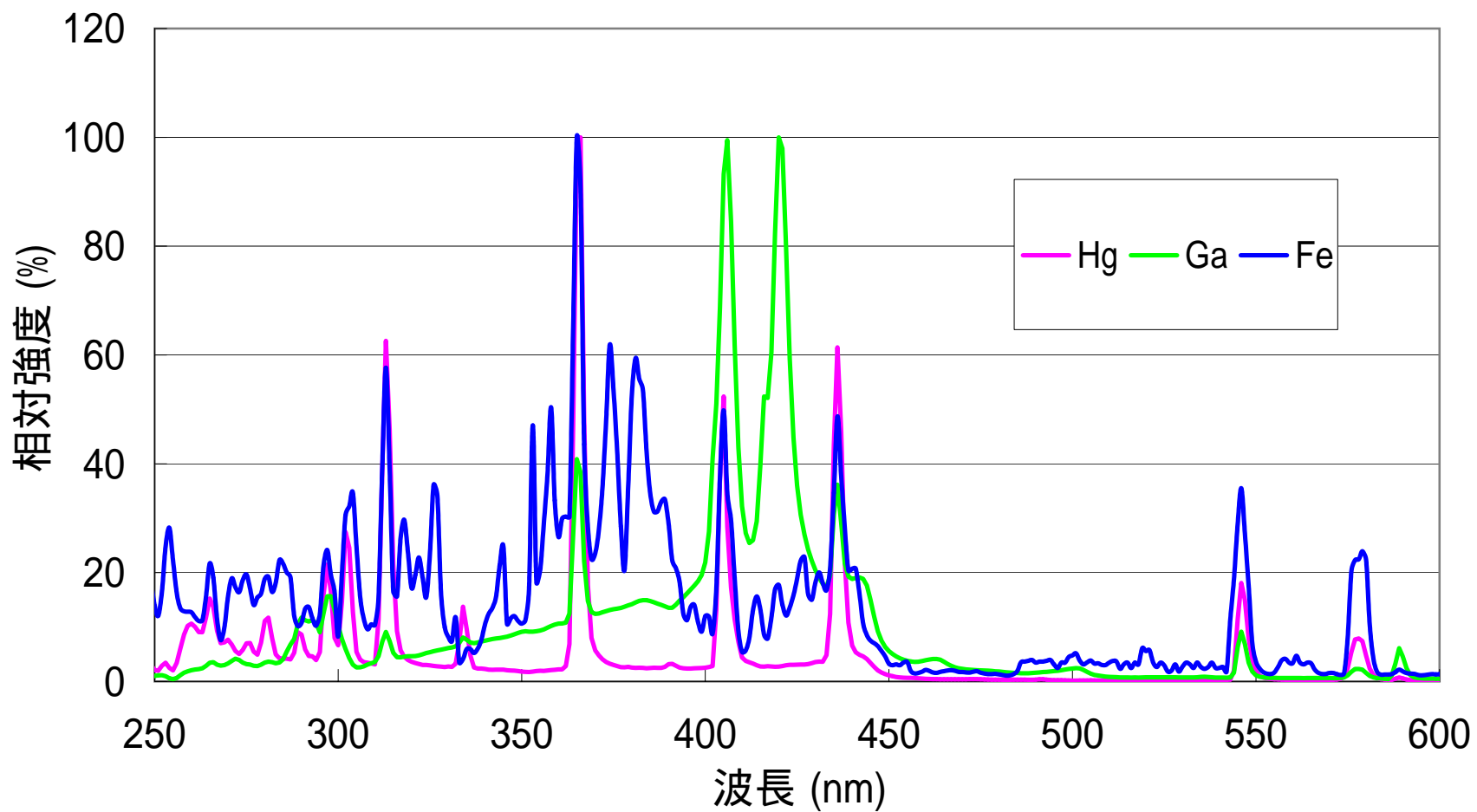
250Wランプ分光分布 (相対強度 (%))
